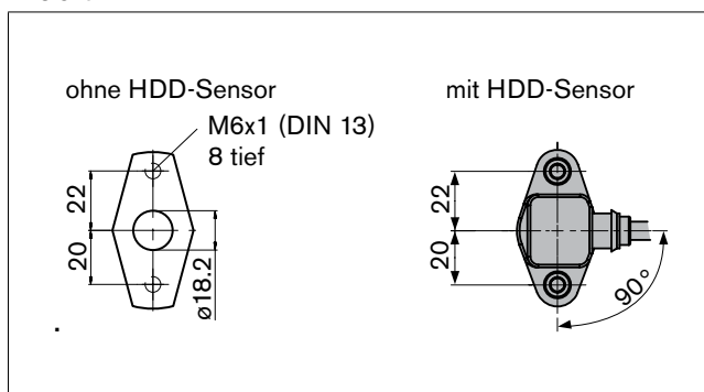
Ansicht X
