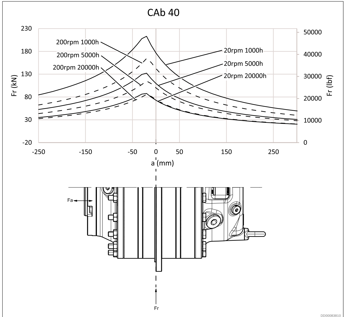
Fig. 35: Permissible external dynamic load Hägglands CAb 40
