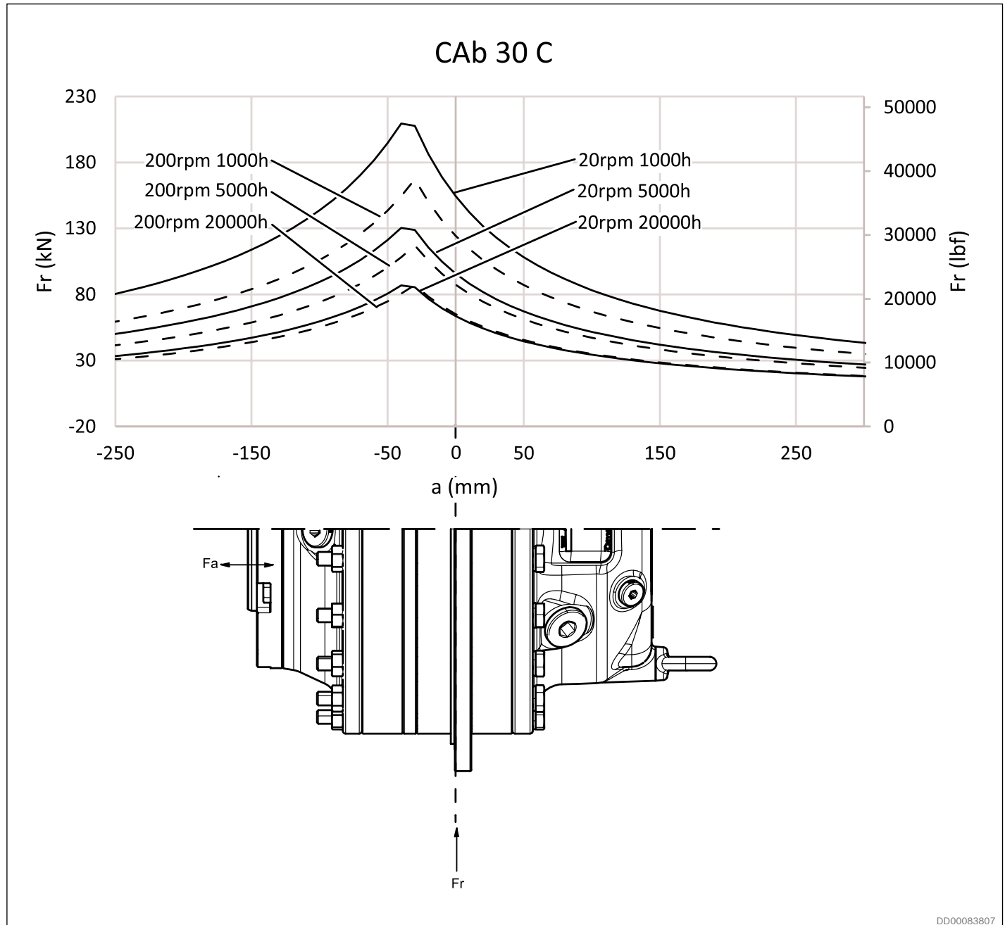
Fig. 33: Permissible external dynamic load Häggblunds CAb 30 C (center flange)
